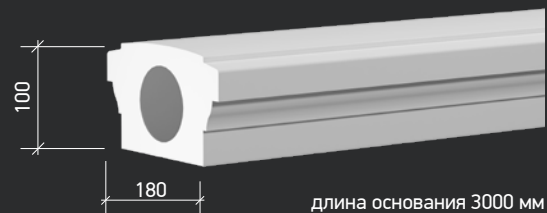
4.79.101 плинтус столба
