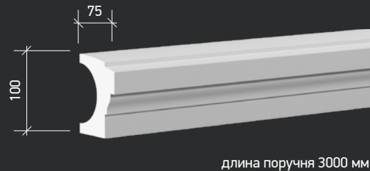
4.72.211 полупоручень
