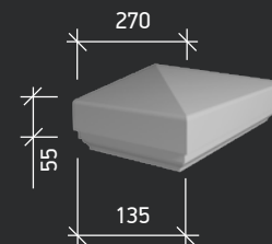
4.76.111 полукрышка пирамида
