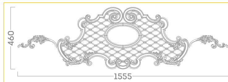
УЗЕЛ 66104BR (460*1555 ММ)
