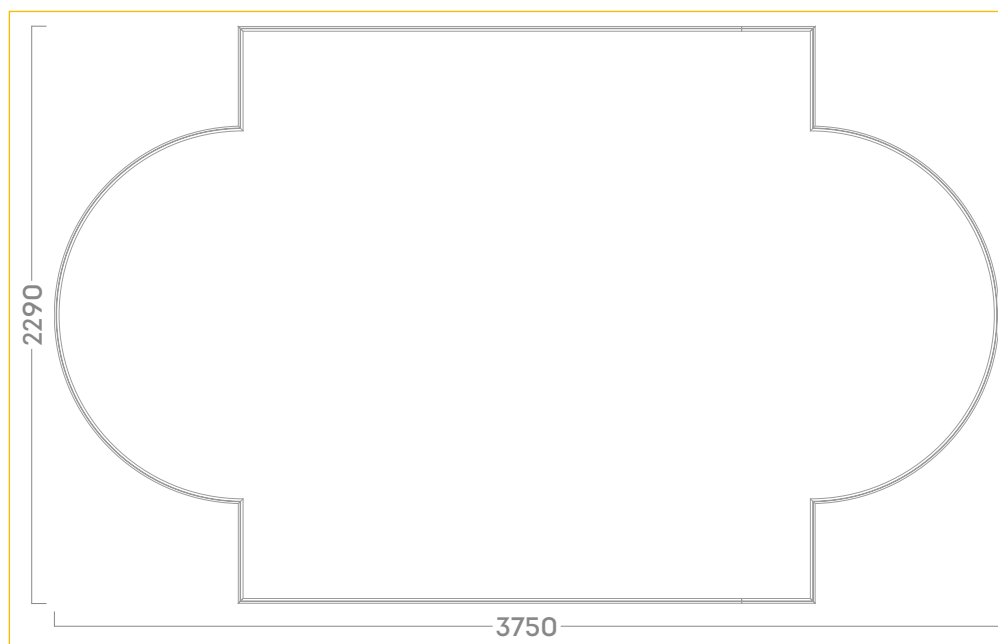
УЗЕЛ 66105BR (2290*3750 ММ)
