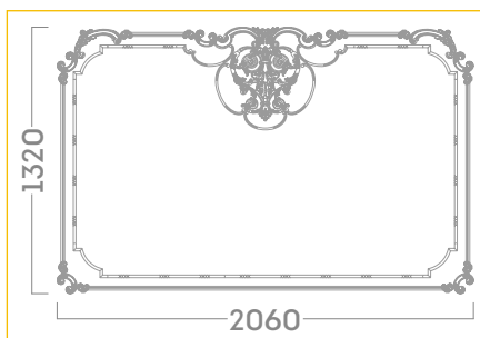
УЗЕЛ 66113BR (1320*2060 ММ)
