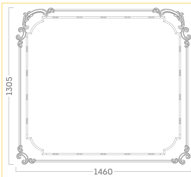
УЗЕЛ 66118BR (1305*1460 ММ)
